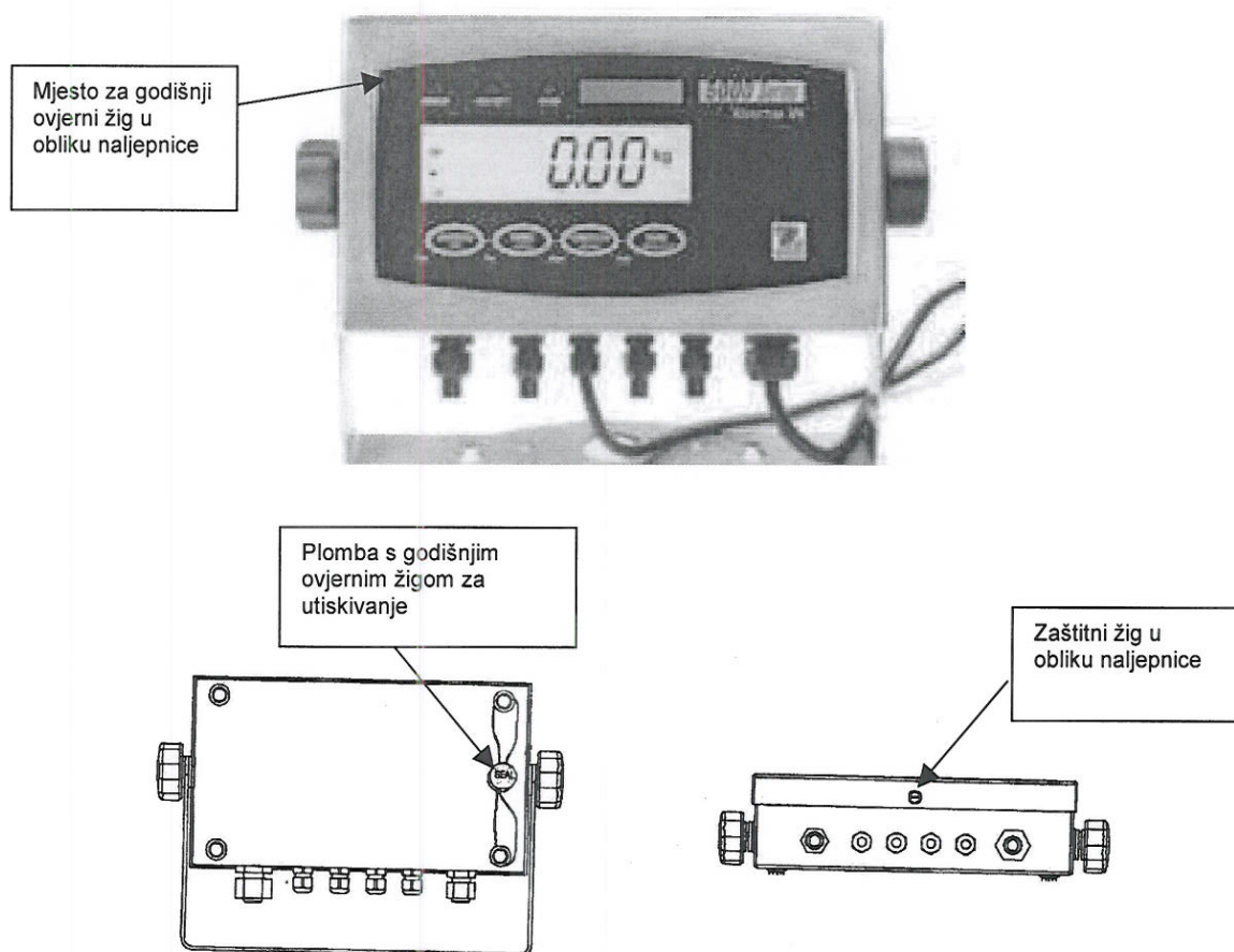
Slika 4: Izgled i način zaštite EPU tipa T51XW
