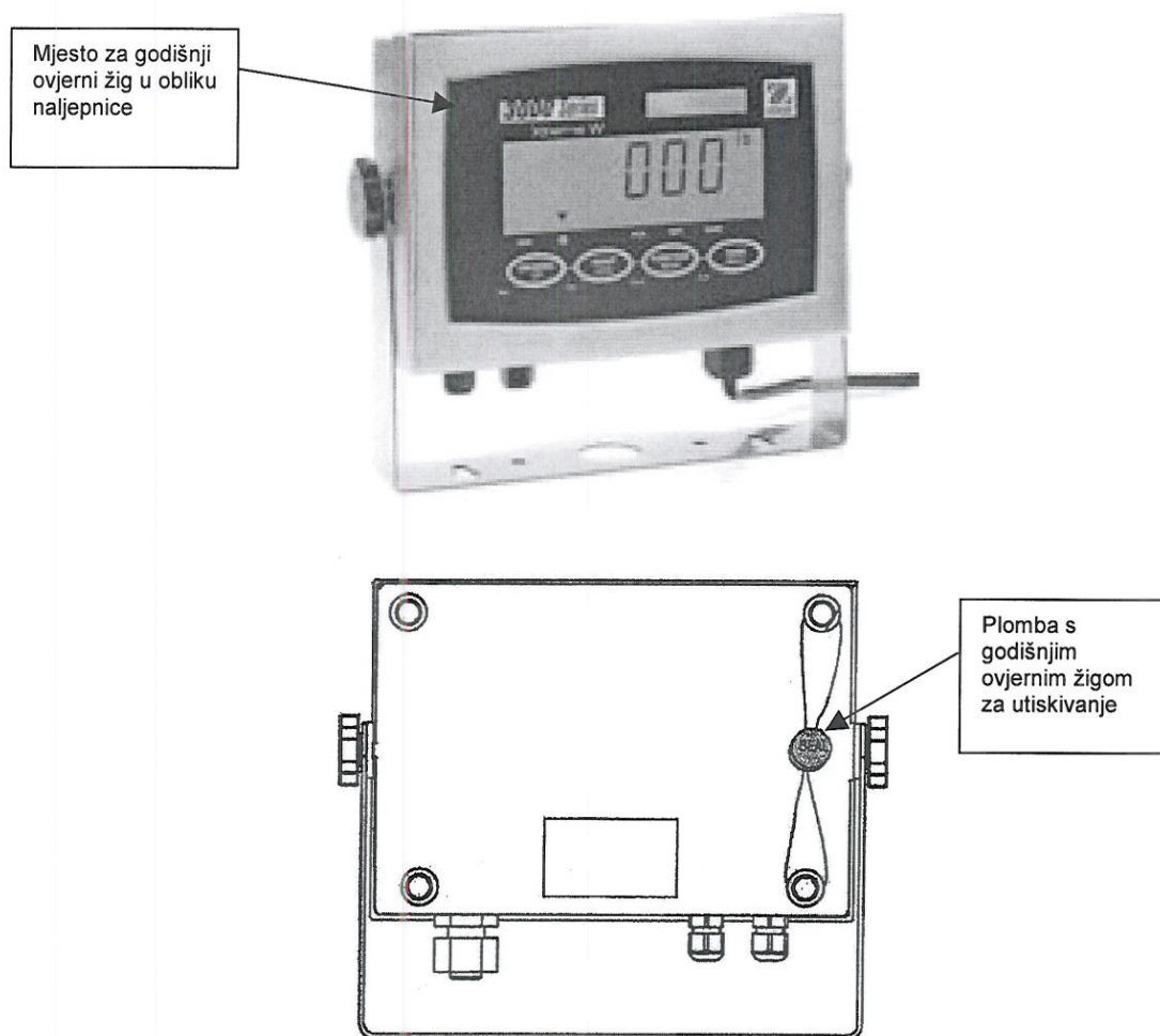
Slika 2: Izgled i način zaštite EPU tipa T31XW
