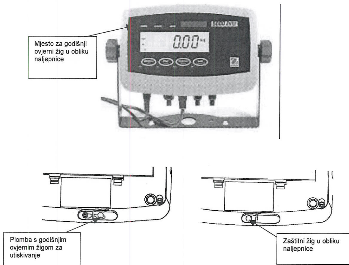
Slika 3: Izgled i način zaštite EPU tipa T51P
